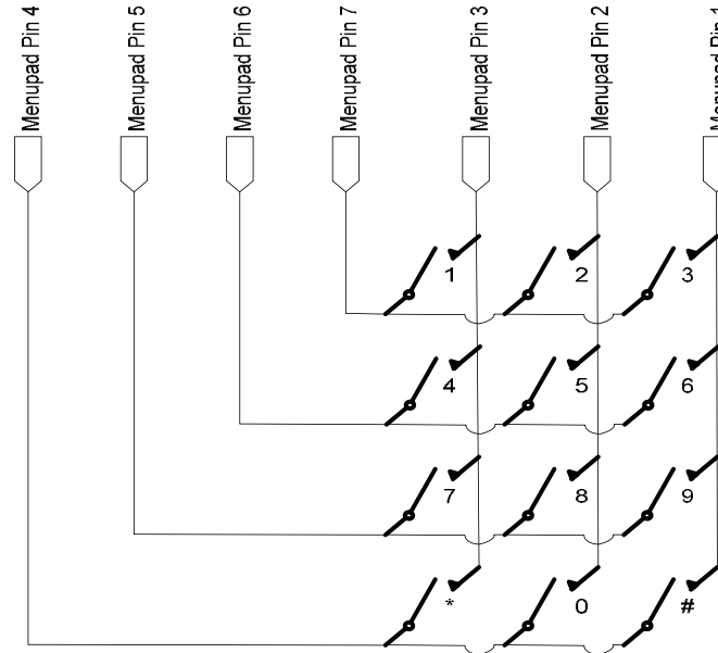
Scan/Matrix Wiring
